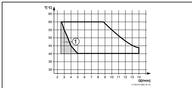
Рис. 12 Диаграмма температуры подаваемой холодной воды от +15 °С (ZWC 28)
